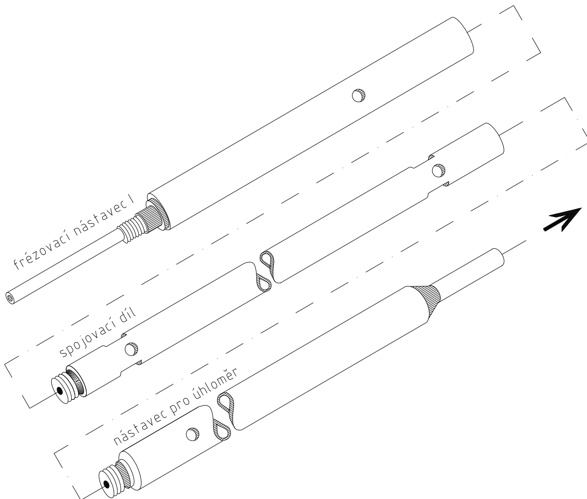
Obr. 18 Sestavený rektifikační trn
