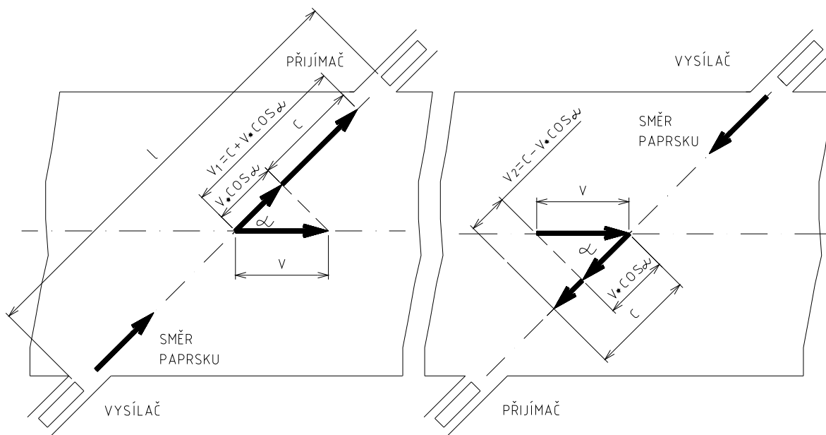
Obr. 1 Princip činnosti
