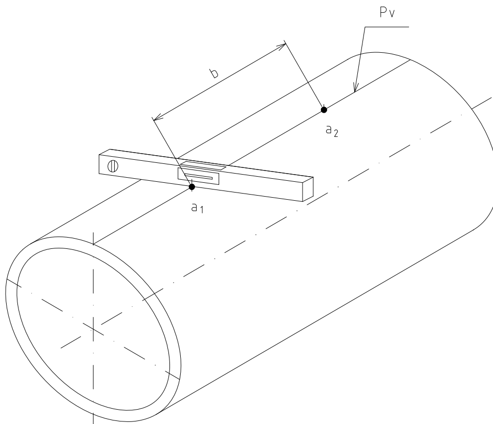
Obr. 14 Vyznačení povrchové vrcholové přímky p_v
