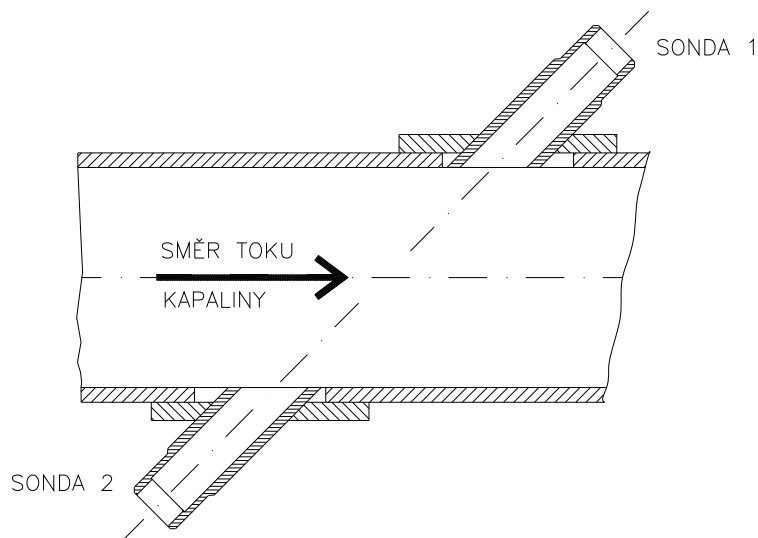
Obr. 24 Označení sond
