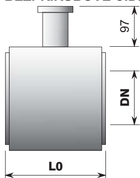
BEZPŘÍRUBOVÉ ČIDLO
