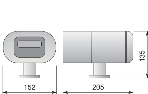
VYHODNOCOVACÍ ELEKTRONIKA
